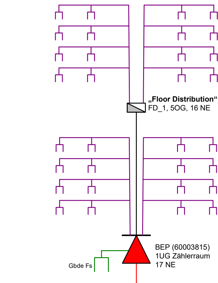
Abbildung 4 Floor Distribution
