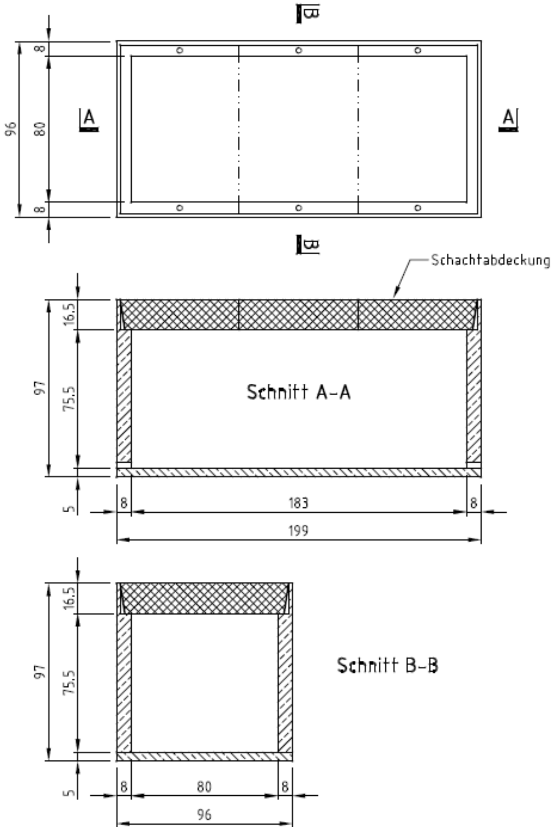
Abbildung 47 LWL-Schacht Kunststoff Langmatz 182.5x80.0 cm
