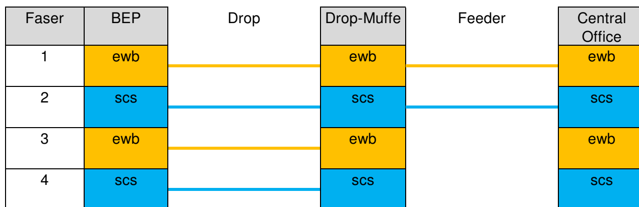
Abbildung 49 Faserbelegung ewb Drop Geschäftskunde
