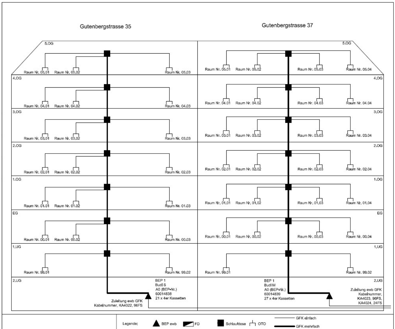
Abbildung 5 OTO mit Flat ID
