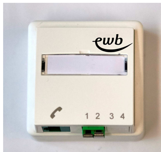
Abbildung 76 Musterbild des Diamond-OTOS mit ewb-Logo
