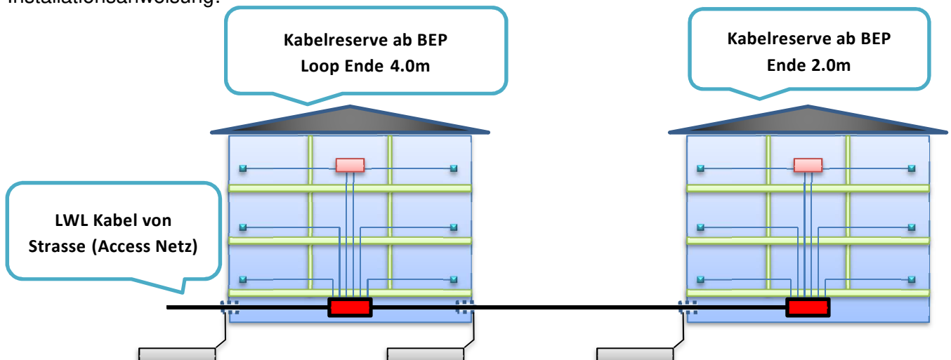
Abbildung 17 Abschlaufung
