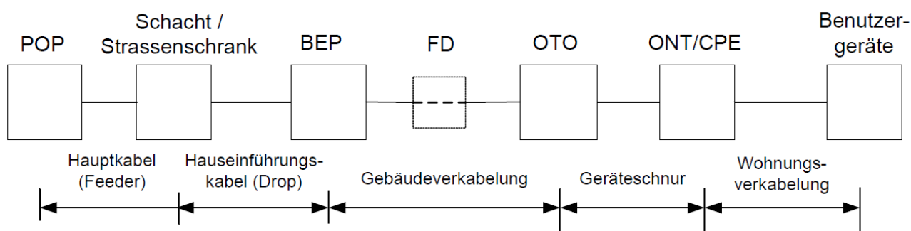
Abbildung 1 Referenzmodell BAKOM
