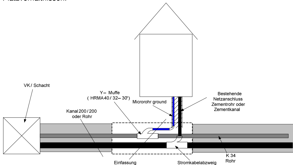
Abbildung 28 Telecomanschluss Variante 4
