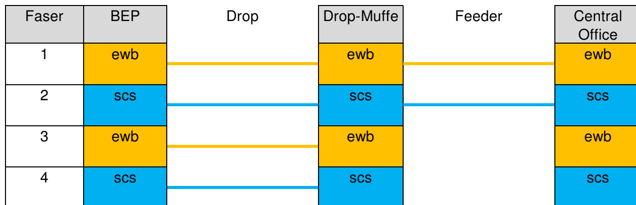
Abbildung 52 Faserbelegung Swisscom Drop Geschäftskunde
