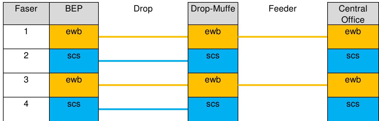
Abbildung 50 Faserbelegung ewb Drop Gebäudefasern
