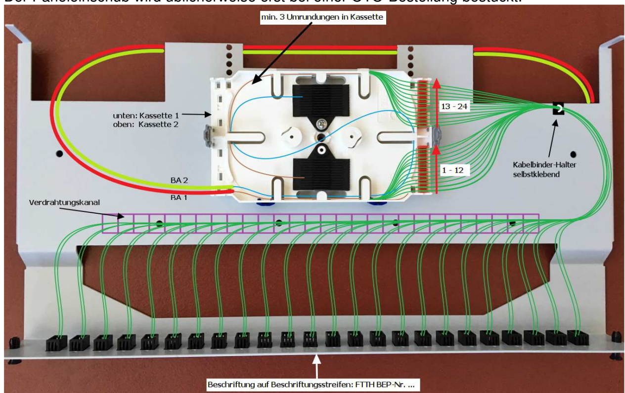
Abbildung 20 Paneleinschub
