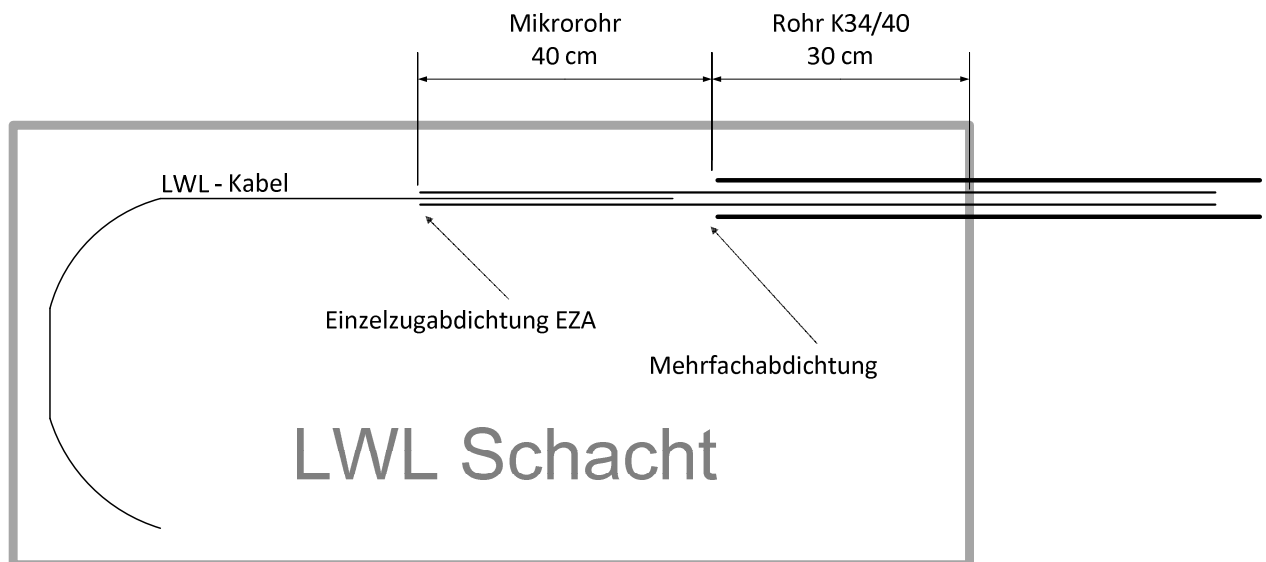
Abbildung 36 Anordnung K34 Rohr im LWL-Schacht
