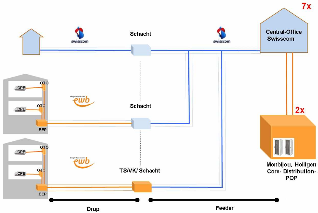
Abbildung 23 Systemarchitektur FTTH
