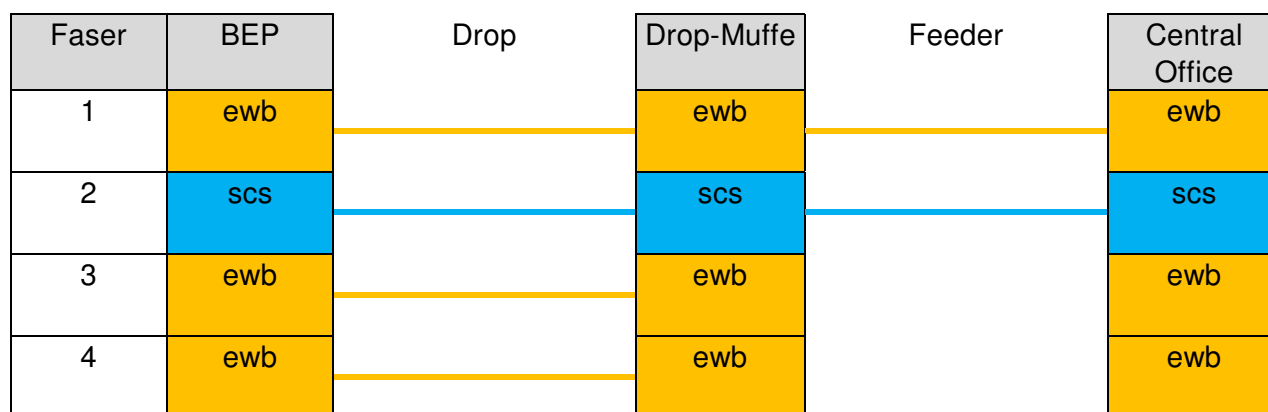
Abbildung 48 Faserbelegung ewb Drop Privatkunde
