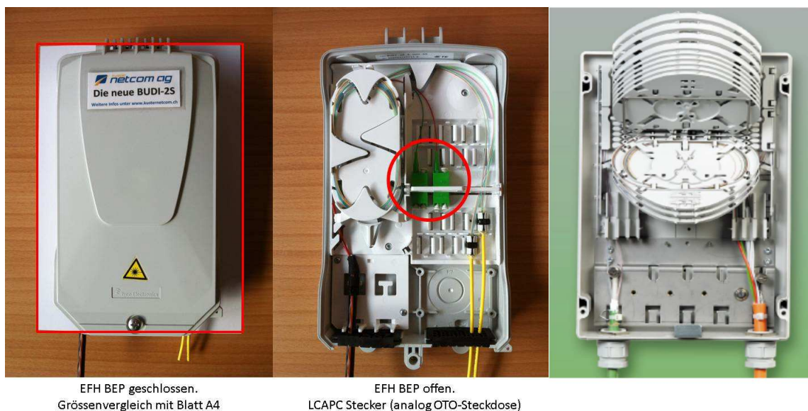
Abbildung 14 EFH BEP
