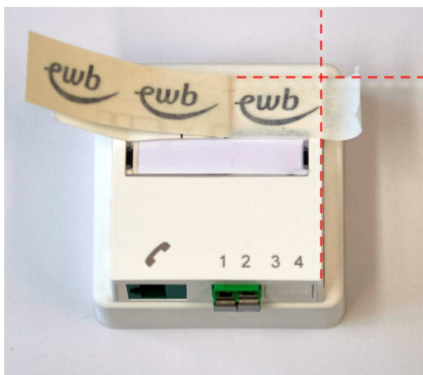
Abbildung 75 Ausrichtung des ewb-Logos auf dem OTO
