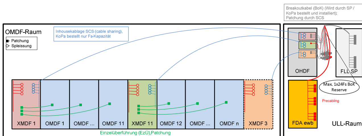
Abbildung 57 Anbindung Aktivausrüstung im CO nach Anschlussvariante 1
