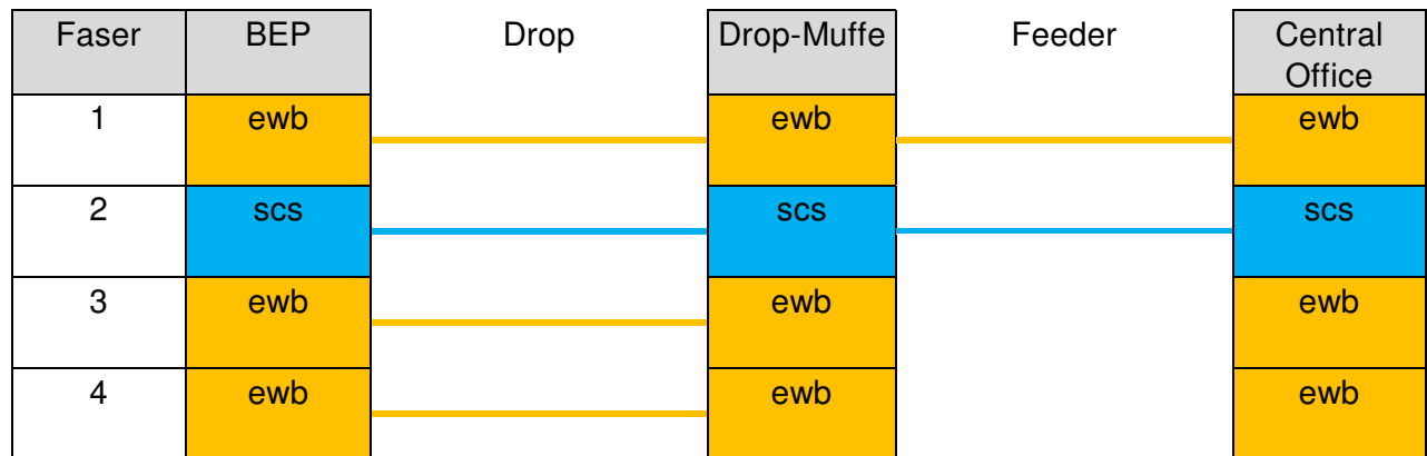
Abbildung 51 Faserbelegung Swisscom Drop Privatkunde
