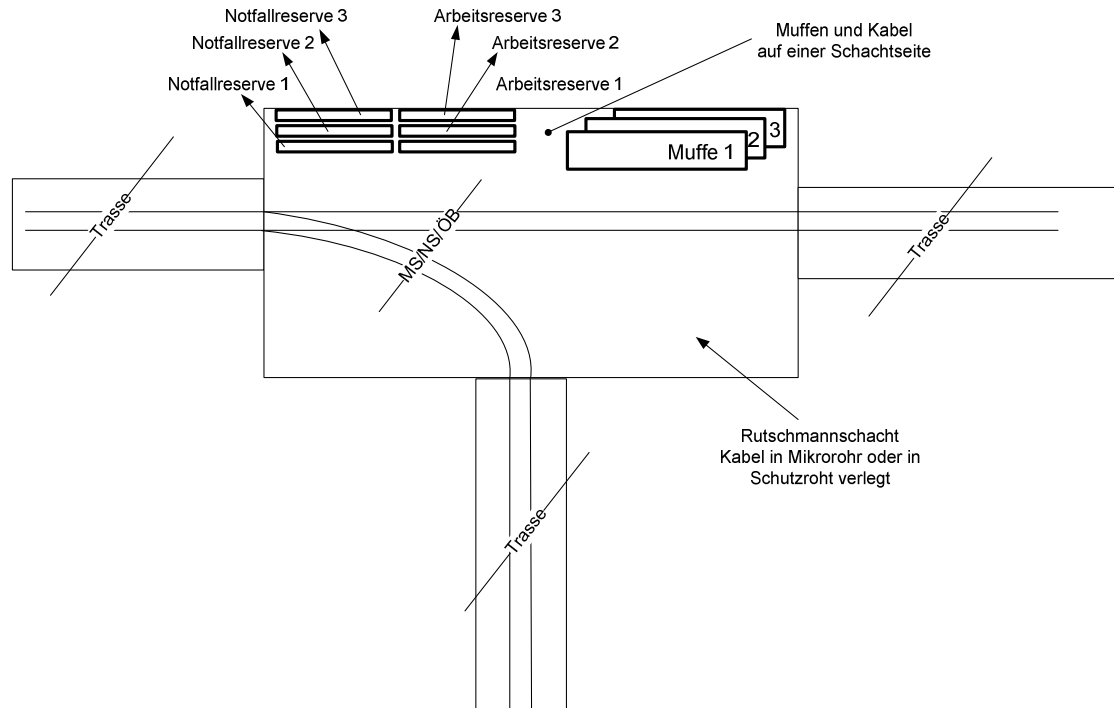
Abbildung 109 Kabelverlegeprinzip Kombischacht
