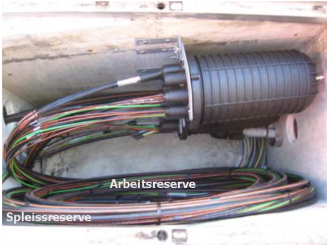
Abbildung 113 Gutes Beispiel Schachtinstallation
