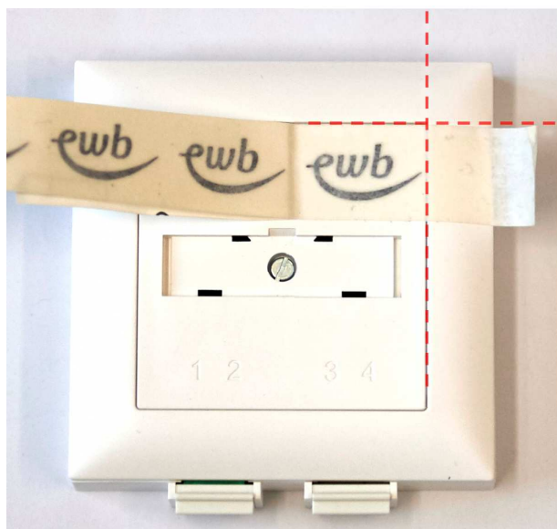
Abbildung 77 Ausrichtung des ewb-Logos auf dem OTO
