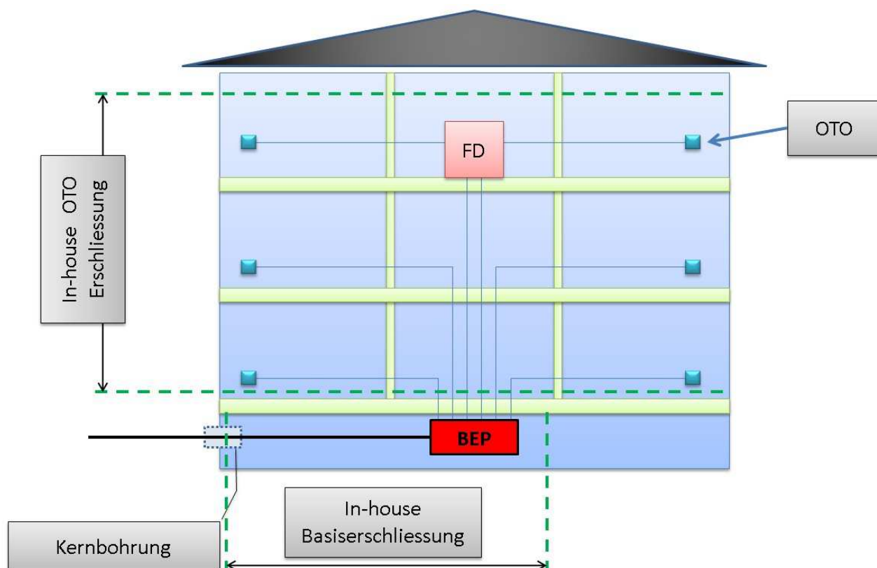
Abbildung 13 Layout Erschliessung Inhouse
