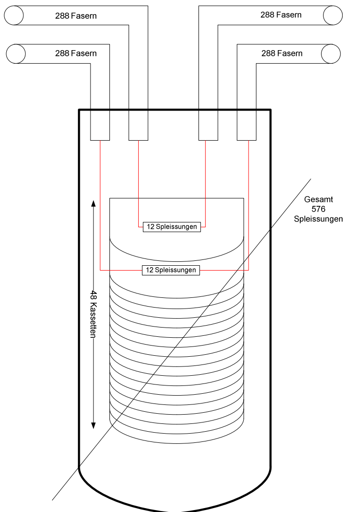
Abbildung 115 Muffenkapazität
