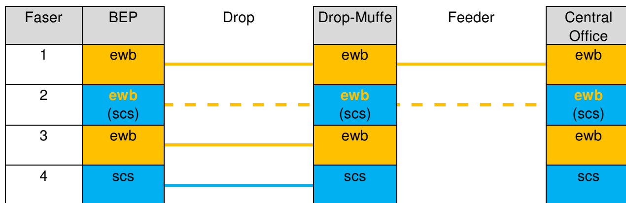
Abbildung 53 Faserbelegung Swisscom Drop Gebäudefasern
