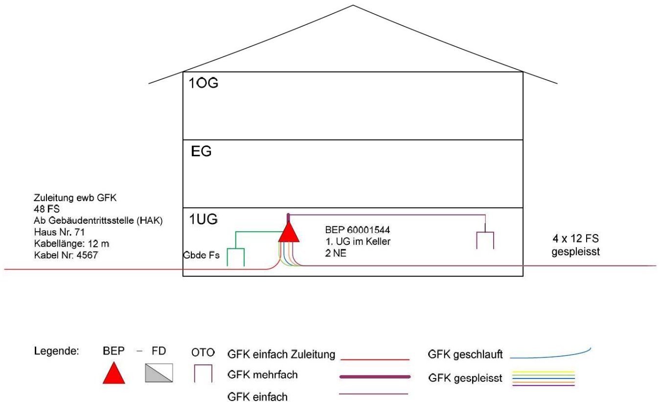
Abbildung 6 Abschlaufung EFH
