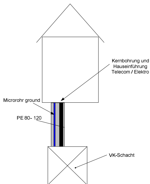
Abbildung 26 Telecomanschluss Variante 2
