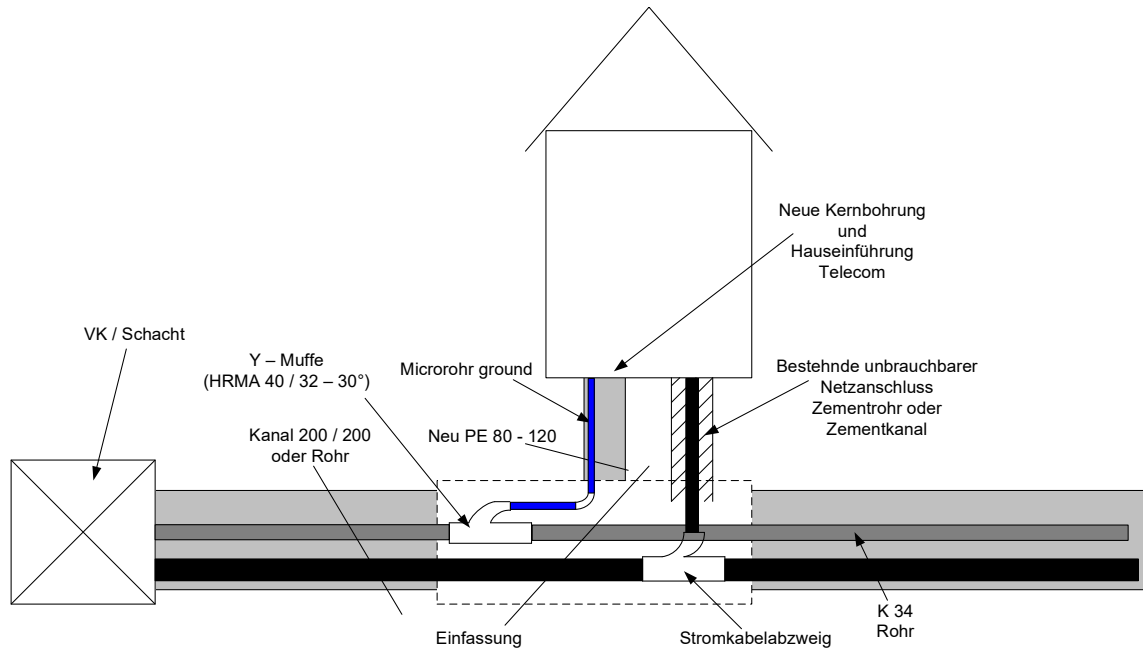
Abbildung 27 Telecomanschluss Variante 3
