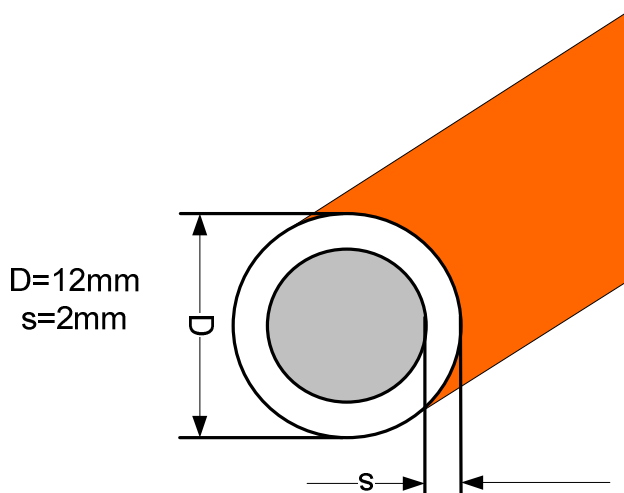
Abbildung 41 Definition Microrohr-Ground
