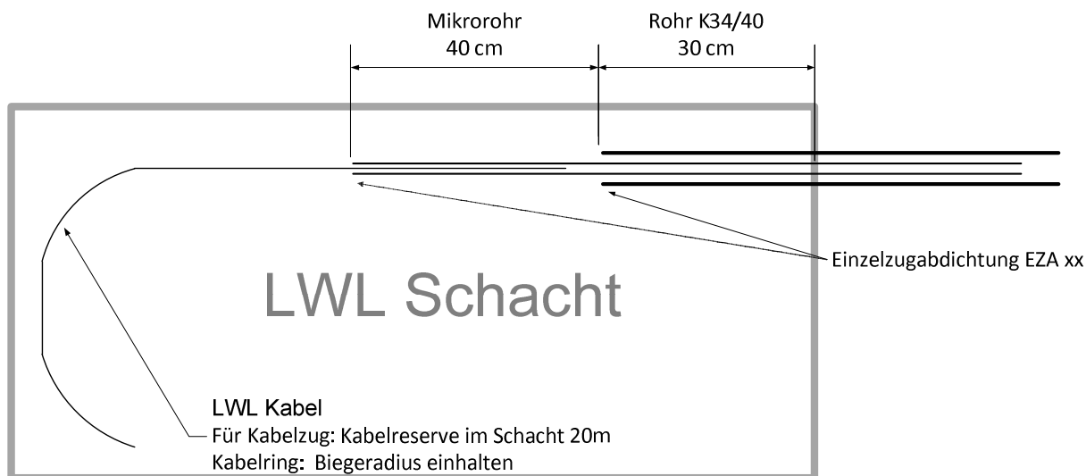
Abbildung 111 Notfallreserve in Schacht
