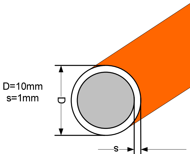
Abbildung 38 Definition Microrohr
