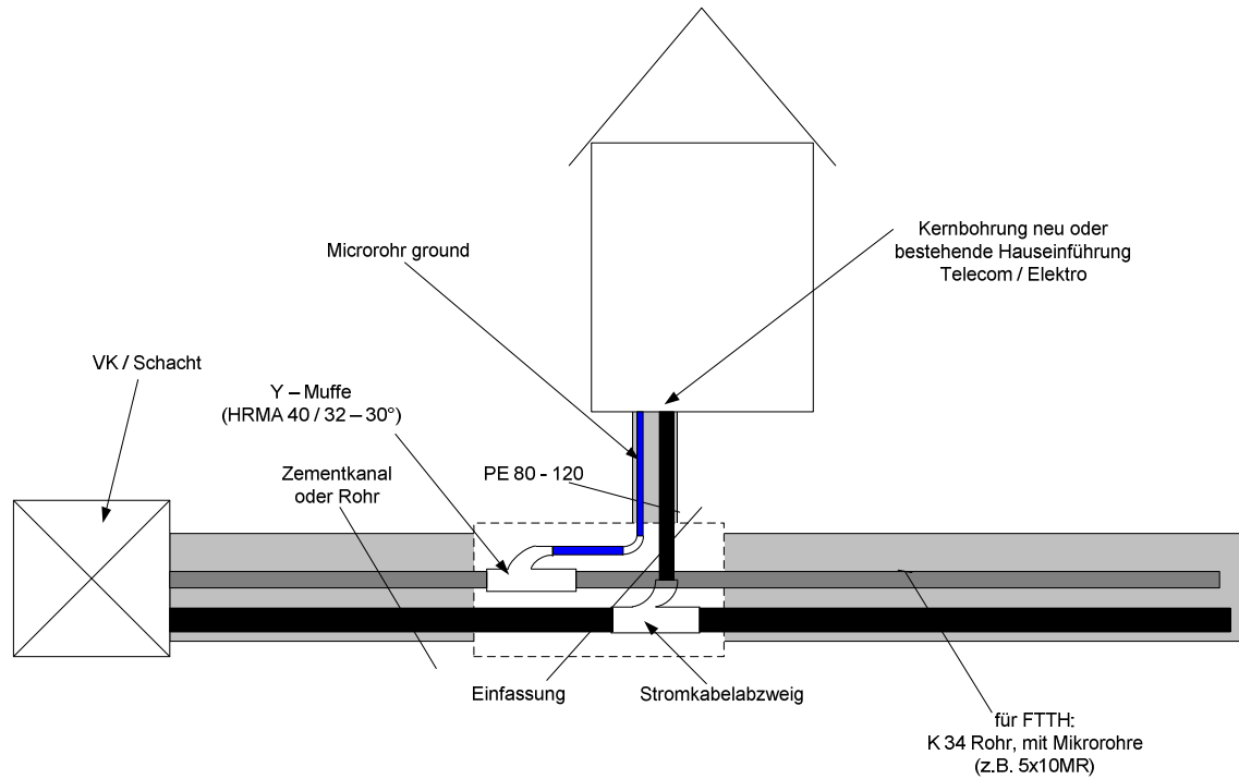
Abbildung 25 Telecomanschluss Variante 1
