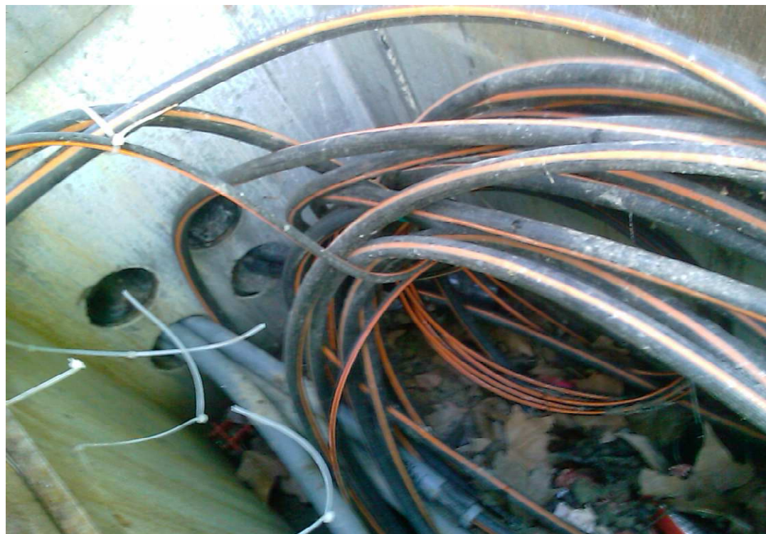
Abbildung 112 Schlechtes Beispiel Schachtinstallation
