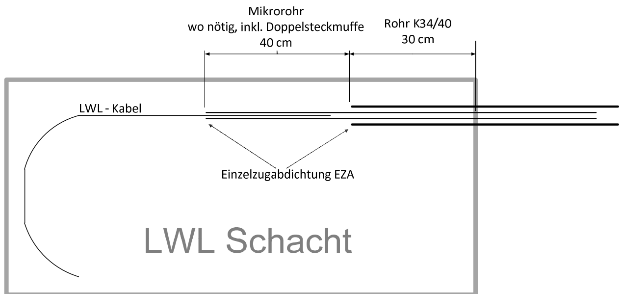
Abbildung 39 Anordnung Microrohr im LWL-Schacht
