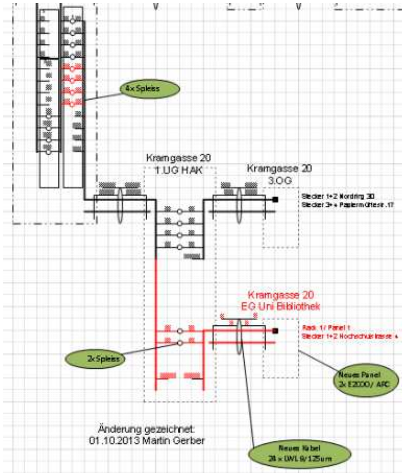
Abbildung 62 Spleissplan
