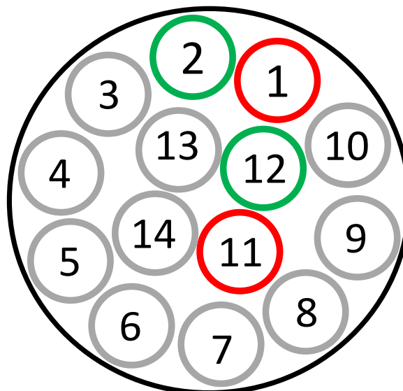
Abbildung 117 Reihenfolge Bündeladern alt, Kabelquerschnitt
