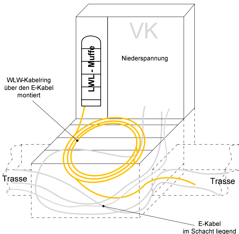
Abbildung 43 Niederspannungs-Verteilerkasten mit separatem Telecomabteil
