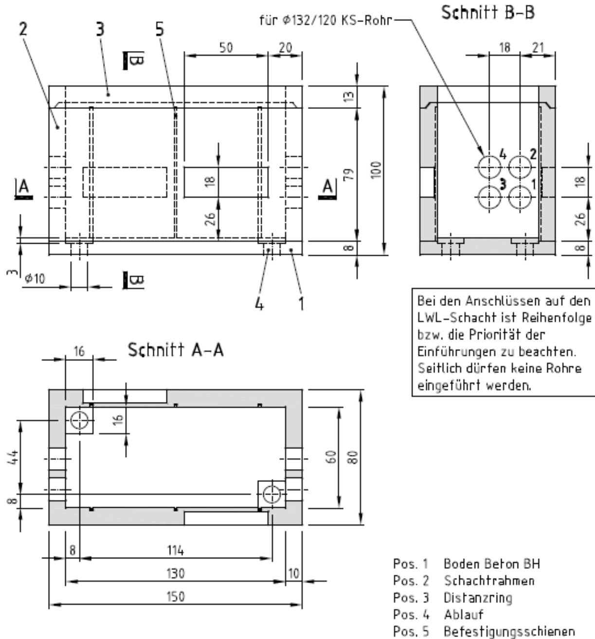
Masse in cm Abbildung 45 LWL-Schacht 130x60 250/400KN
