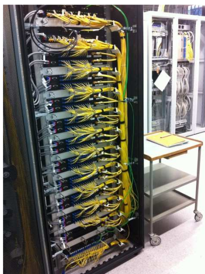
Abbildung 65 Erstes Rack, Frontansicht, CO BOL
