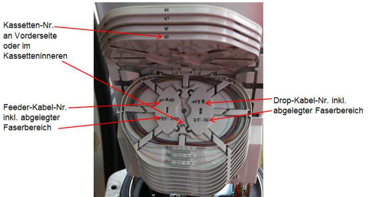
Abbildung 88 Muffen-Spleisskassetten inkl. Beschriftung
