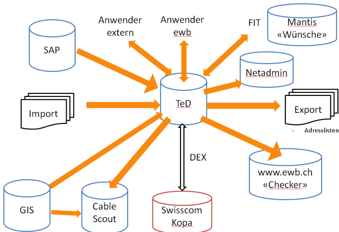
Abbildung 122 Systemlandschaft
