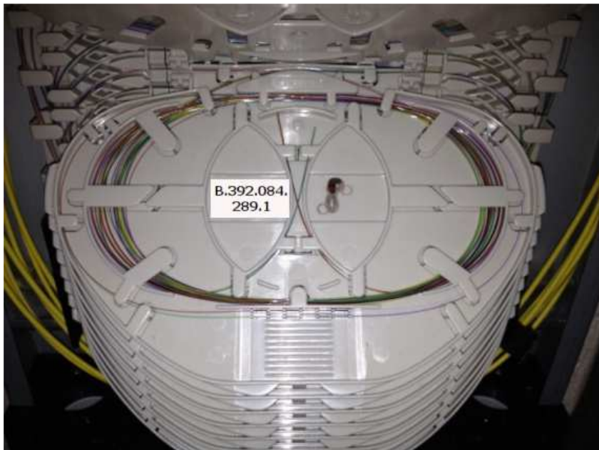
Abbildung 83 BEP Kassette inkl. Beschriftung
