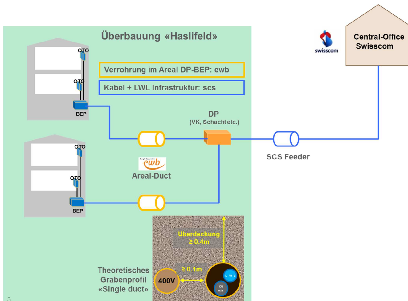
Abbildung 29 Prinziperschliessung Neubauten - Single Duct
