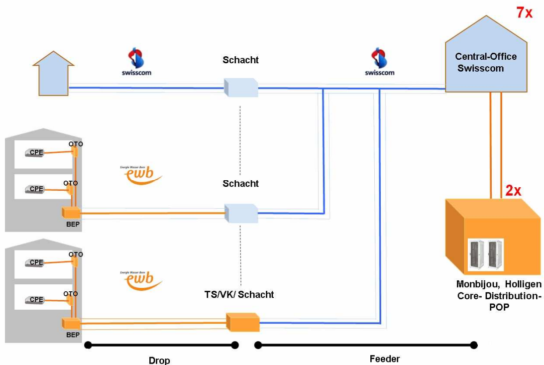
Abbildung 54 Prinzip Berner Glasfasernetz
