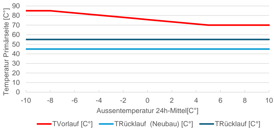
Abbildung 1: Wärmeverbund Neufeld, Viererfeld, Tiefenau, primärseitige Temperaturen
