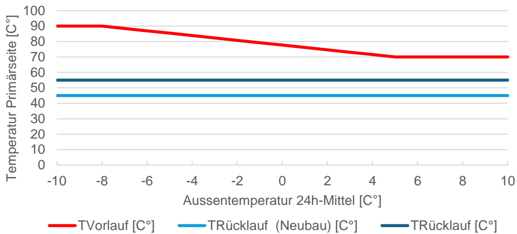
Abbildung 1: Wärmeverbund Bern West, primärseitige Temperaturen
